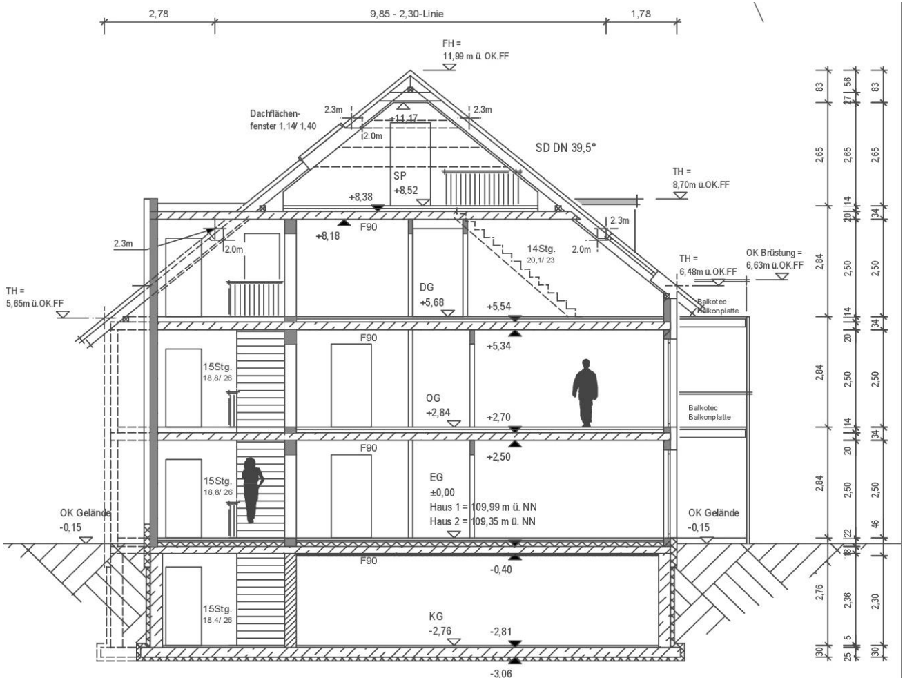
Schnitt
